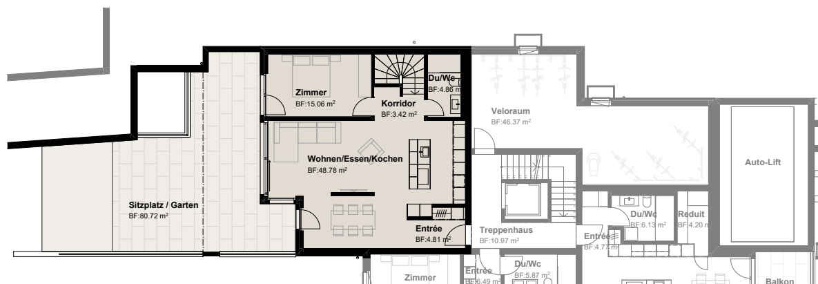
Grundriss Erdgeschoss
