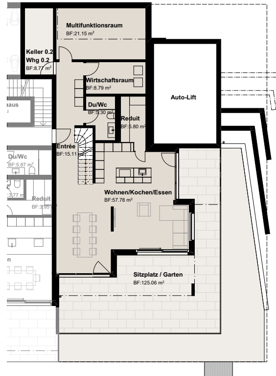
Grundriss Gartengeschoß
